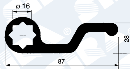
PROFILO TENSIONATORE
