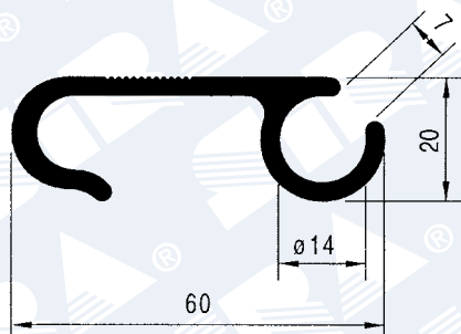
PROFILO AGGANCIAMENTO TELO
