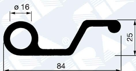
PROFILO TENSIONATORE
