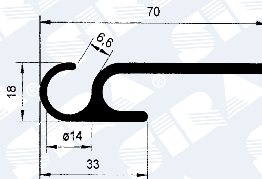
PROFILO AGGANCIAMENTO TELO
